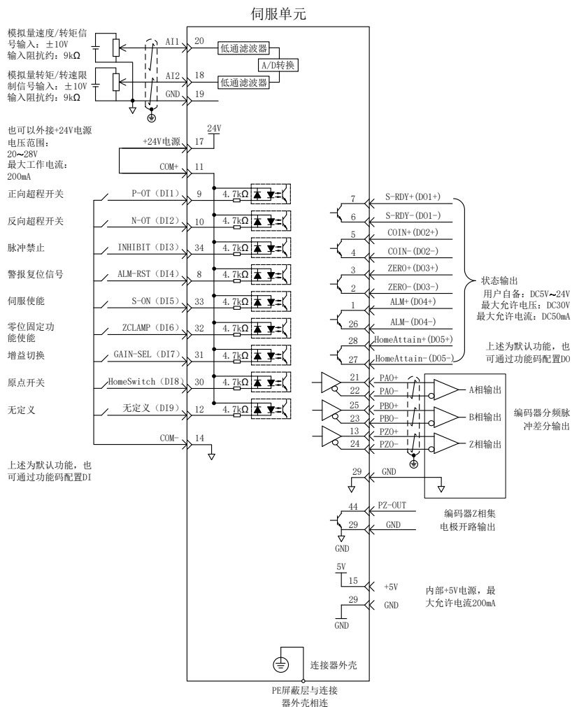
图 4-6 转矩模式配线图
