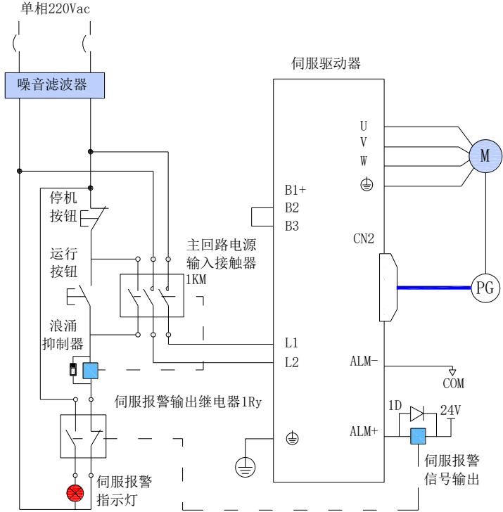
图 3-1 单相 220V 主电路配线
